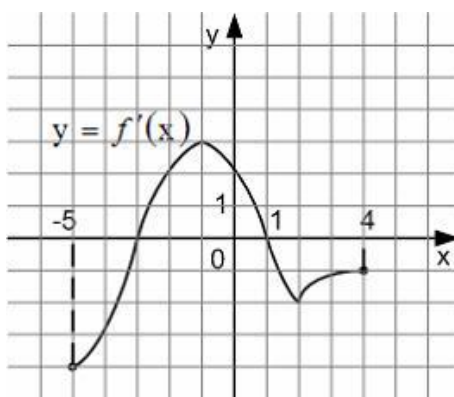
Рисунок. График производной функции y = f'(x)
